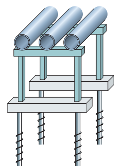
配管等の軽量設備
