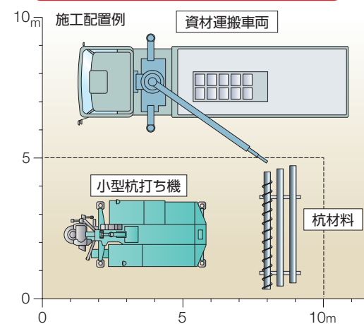
小型杭打ち機
