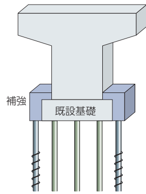
基礎補強 (増し杭)
